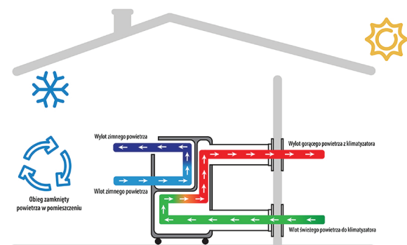
KLIMATYZATOR W POMIESZCZENIU OPCJA Z ADAPTEREM PLENUM OBIEGU GÓRĄCEGO POWIETRZA WZROST EFEKTYWNOŚCI O 60%
