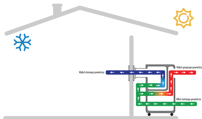
KLIMATYZATOR NA ZEWNĄTRZ POMIESZCZENIA INSTALACJA Z JEDNĄ RURĄ WLOTOWĄ
