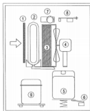
Urządzenie posiadające zbiornik z wyłącznikiem wagowym
